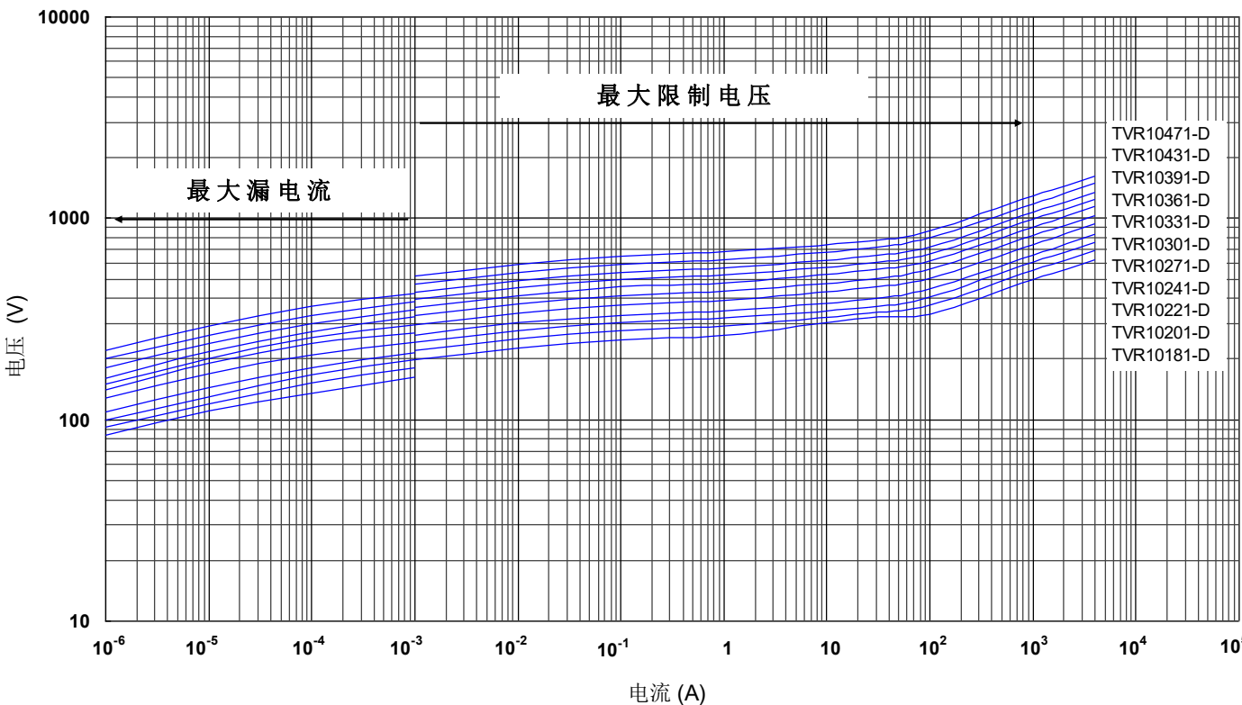
最大漏电流与最大限制电压曲线 (TVR10181-D to TVR10471-D)
