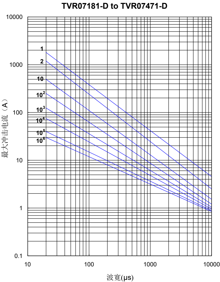
最大冲击电流减额曲线
