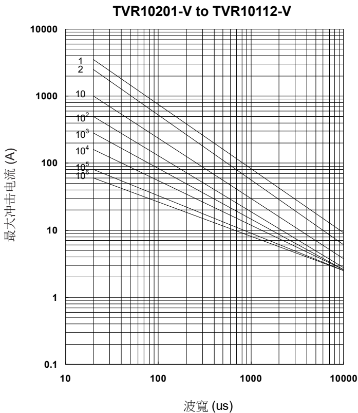
最大冲击电流减额曲线
